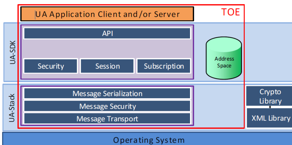
Figure 1 - Architecture Produit.
