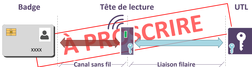
FIGURE 15 – Configuration type n°3: Badge non sécurisé, avec chiffrement filaire seulement
