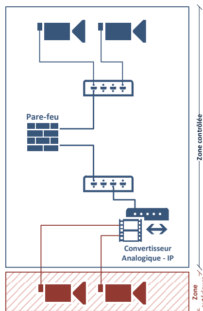
FIGURE 6 – Exemple recommandé de réseau support dédié aux caméras extérieures
