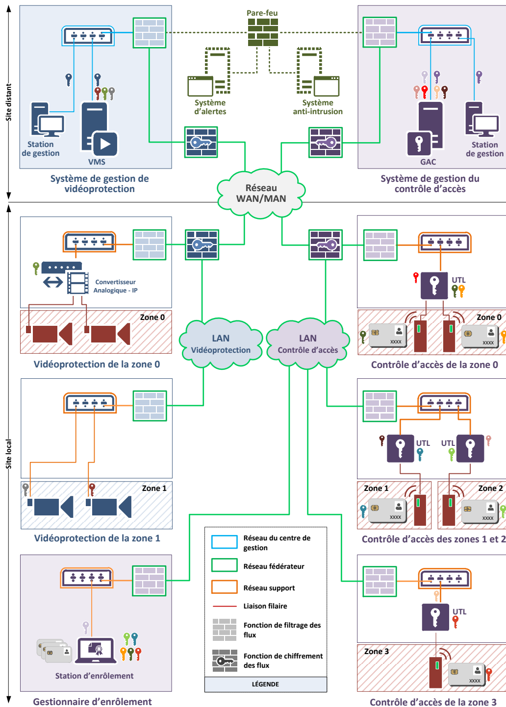
FIGURE 1 – Exemple d'architecture générale
