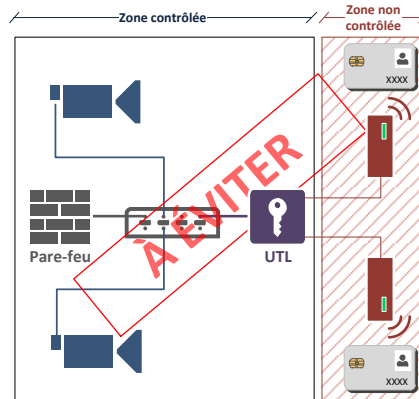
FIGURE 4 – Exemple à éviter de mutualisation du réseau support
