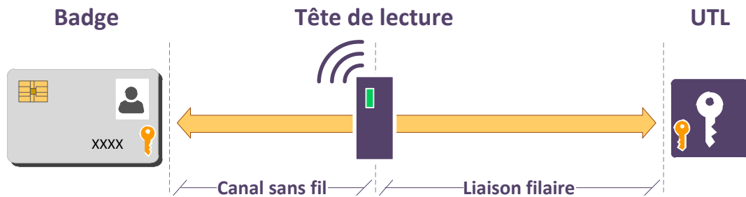
FIGURE 13 – Configuration type n°1 : tête de lecture transparente, authentification de bout en bout
