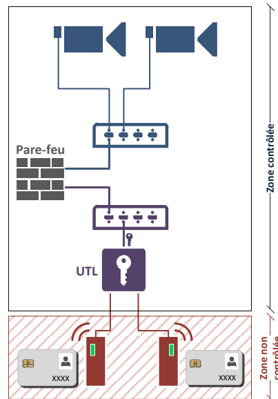
FIGURE 5 – Exemple recommandé de réseaux support non mutualisés
