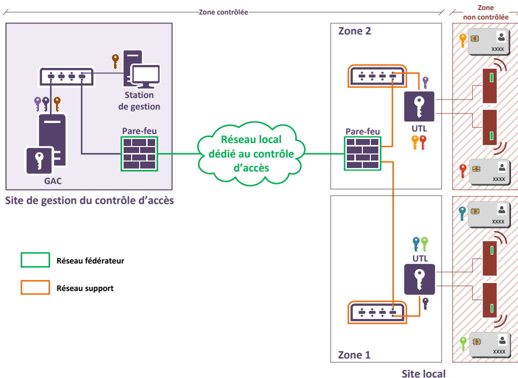
FIGURE 7 – Exemple d'architecture incluant plusieurs réseaux support
