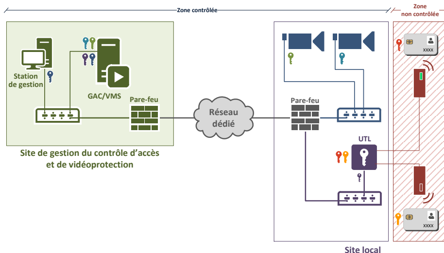
FIGURE 11 – Exemple de mutualisation des fonctions de gestion sur un seul serveur
