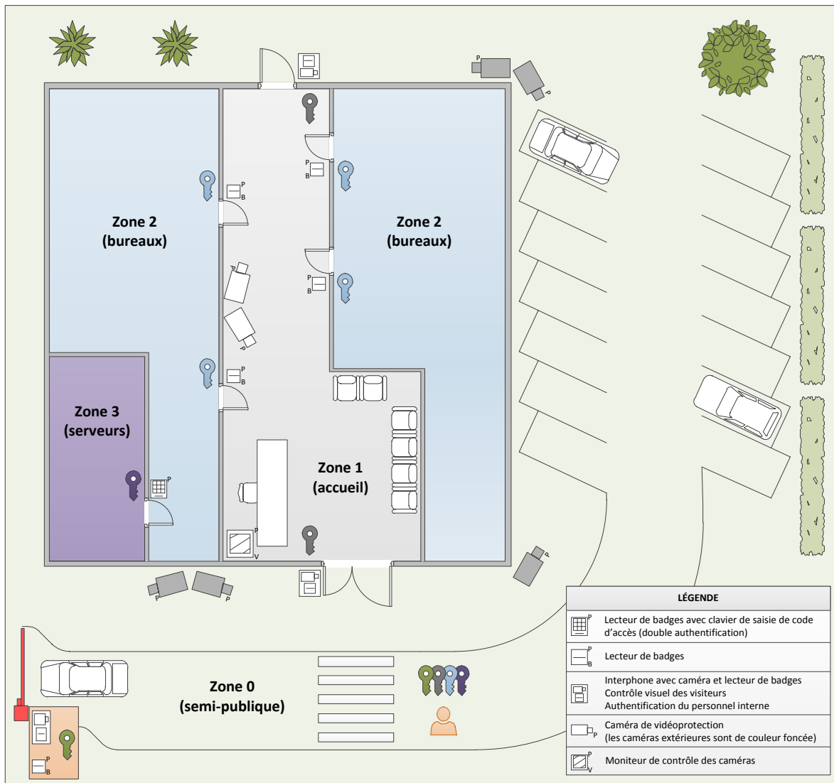
FIGURE 18 – Différenciation des clés utilisées selon le niveau de protection attendu des zones
