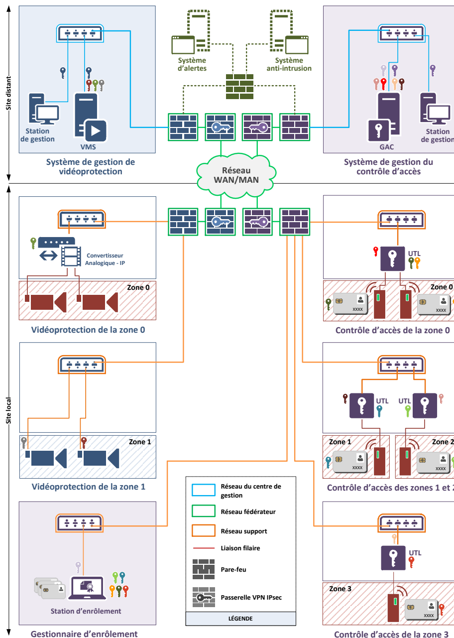
FIGURE 22 – Schéma d'architecture
