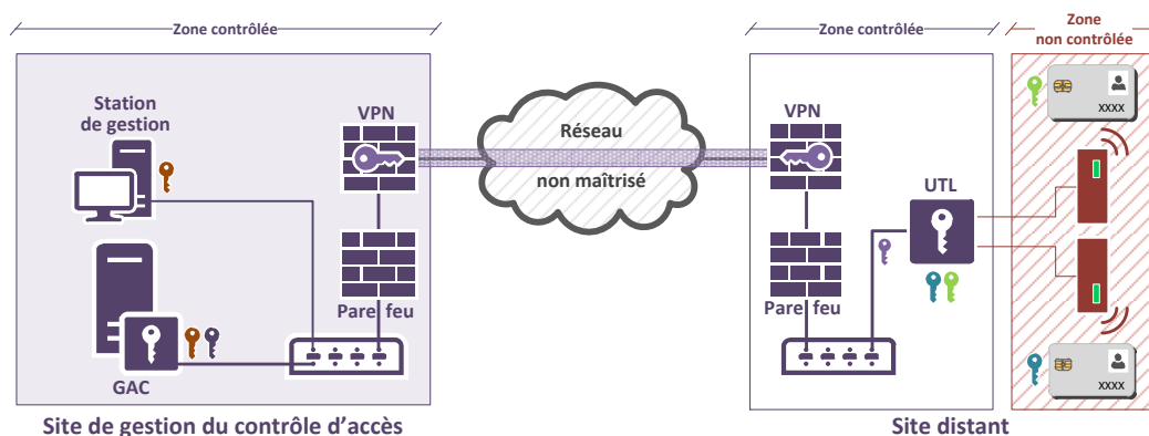
FIGURE 8 – Exemple de réseau fédérateur reposant sur un réseau de transport non maîtrisé
