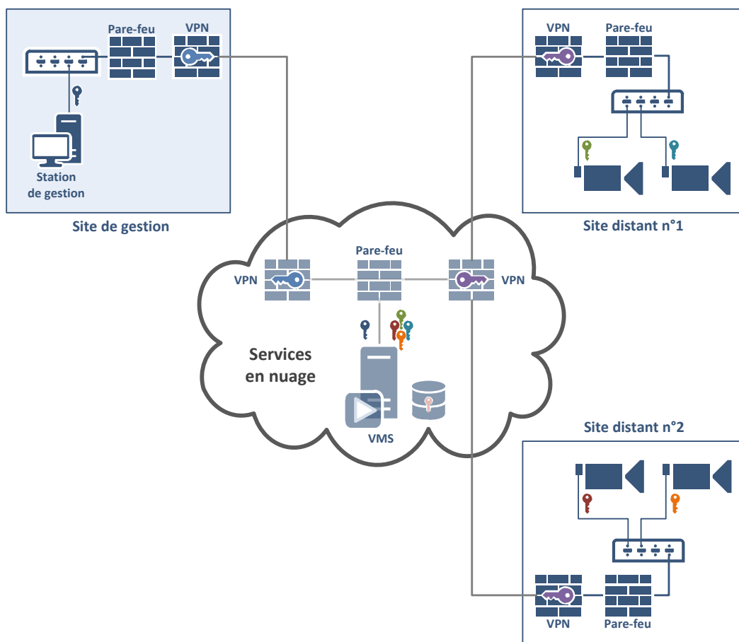
FIGURE 9 – Exemple d’architecture incluant l’hébergement du serveur de gestion de vidéoprotection sur un service d’informatique en nuage
