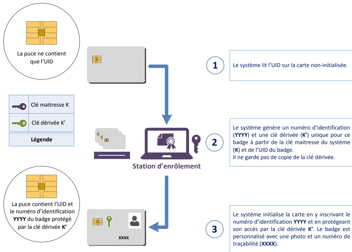
FIGURE 17 – Processus d'initialisation des badges à clé symétrique dérivée
