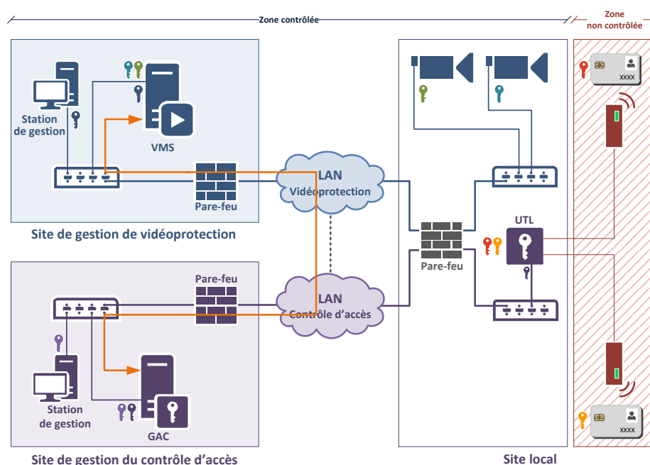
FIGURE 10 – Exemple d'interconnexion entre deux serveurs de gestion
