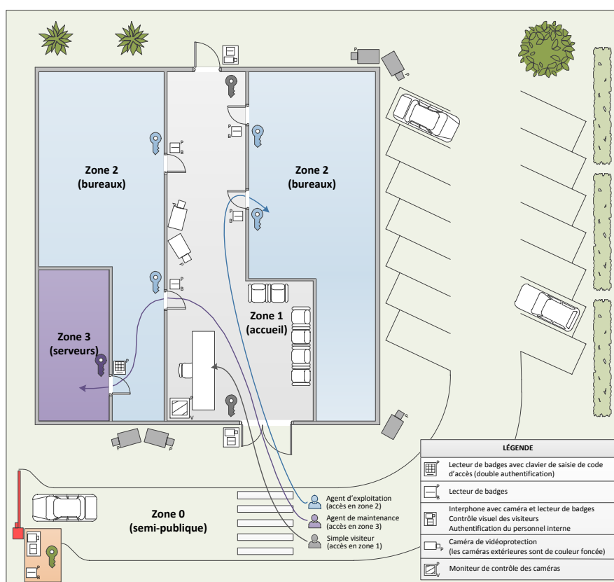
FIGURE 21 – Découpage du site local en zones
