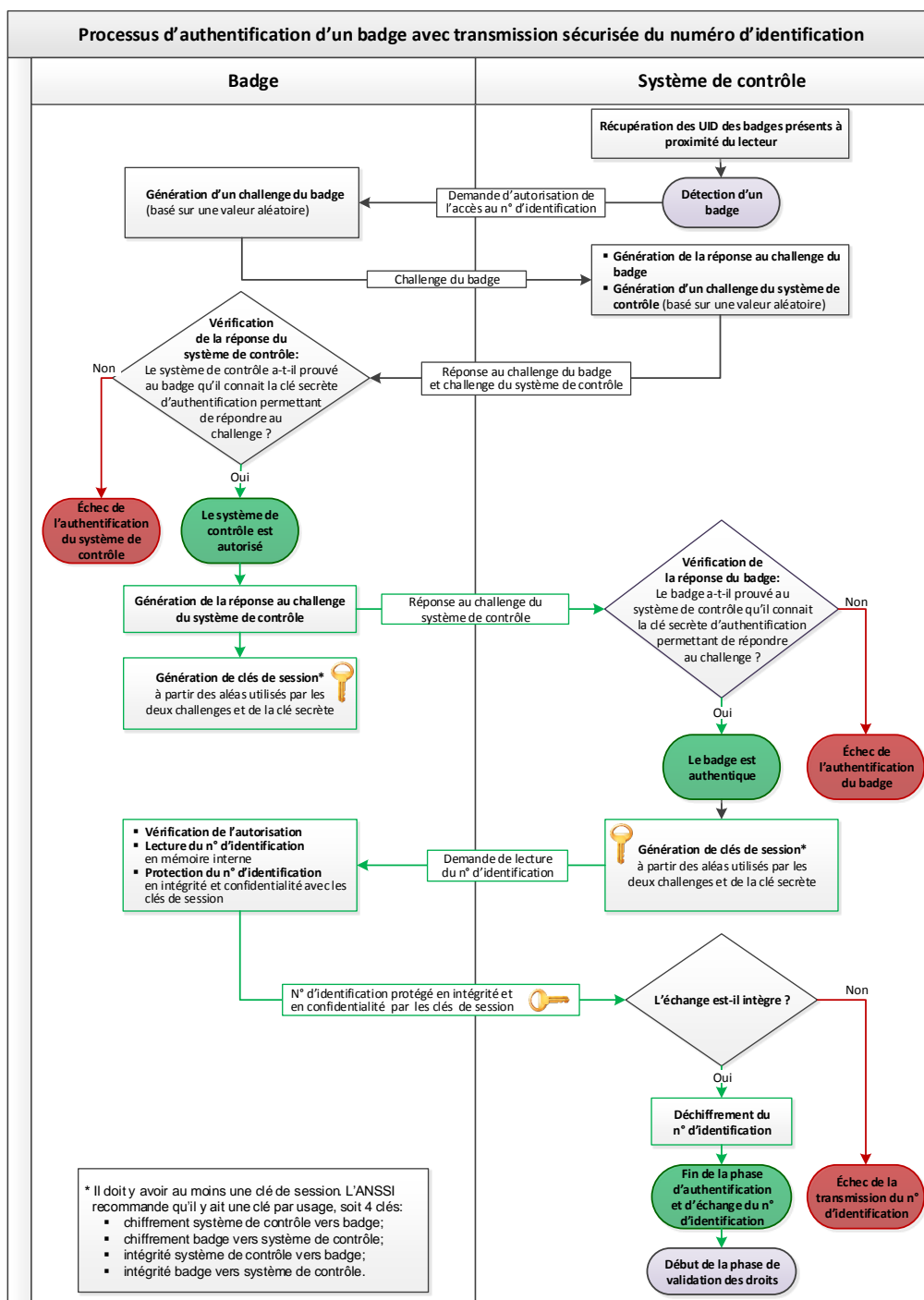
FIGURE 19 – Authentification d'un badge et transmission sécurisée du numéro d'identification
