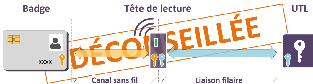
FIGURE 14 – Configuration type n°2: tête de lecture intelligente, double authentification en coupure
