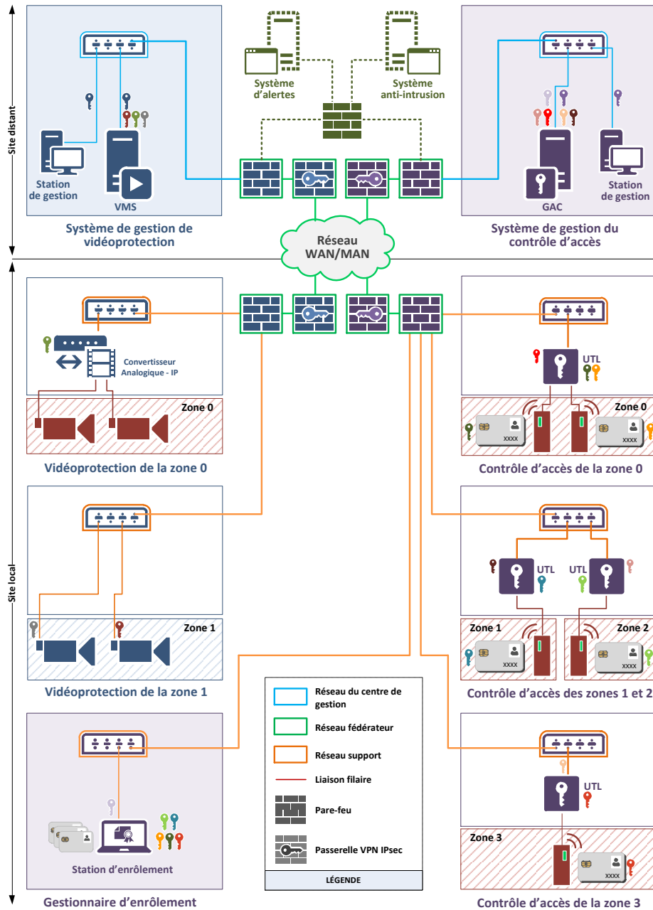
FIGURE 25 – Schéma d'architecture
