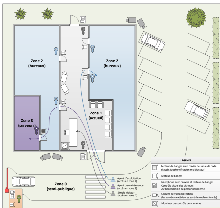
FIGURE 24 – Découpage du site local en zones
