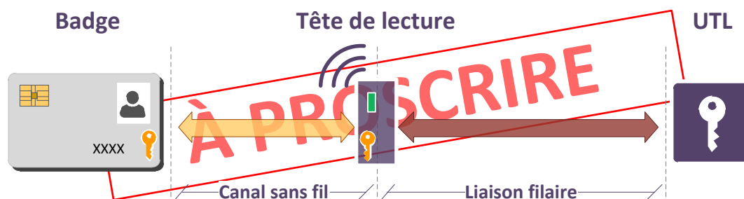
FIGURE 17 – Configuration type n°4 : Badge sécurisé, avec liaison filaire non chiffrée
