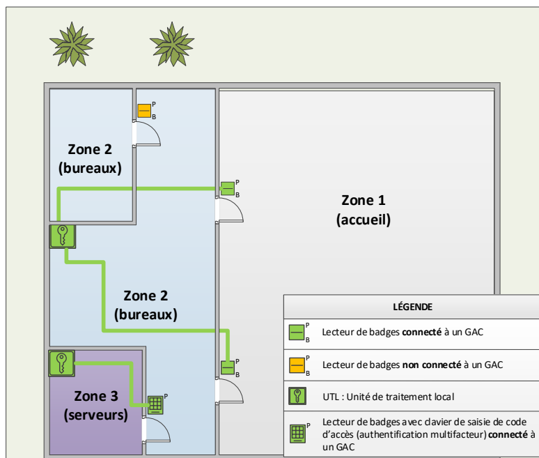
FIGURE 18 – Exemple d'architecture avec un contrôle d'accès physique sans gestion centralisée
