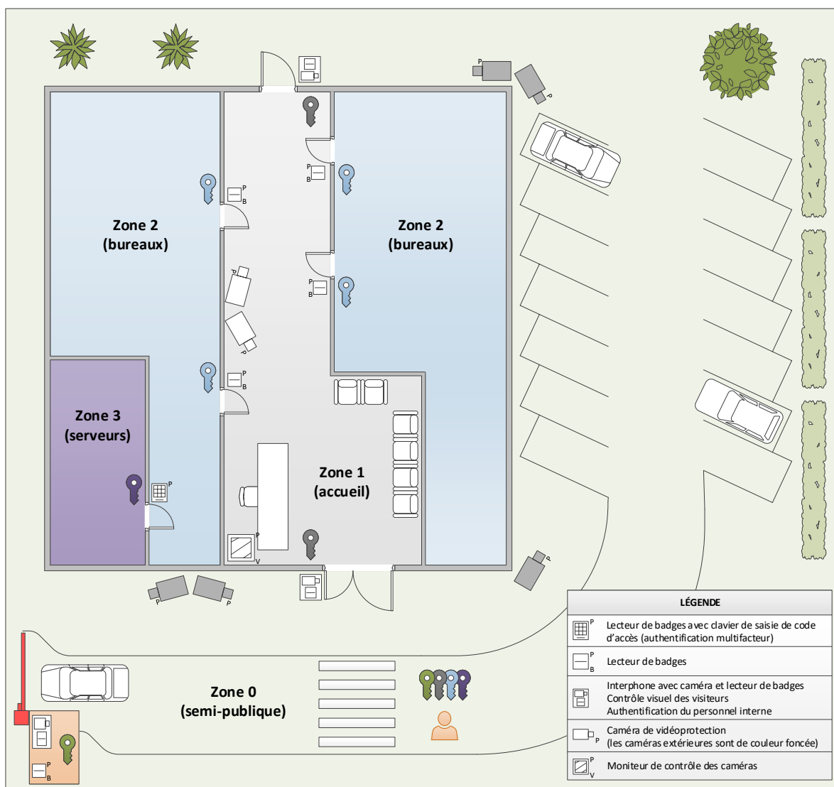
FIGURE 21 – Différenciation des clés utilisées selon le niveau de protection attendu des zones
