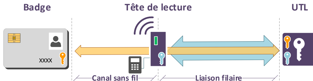
FIGURE 14 – Configuration type n°1 avec introduction d'un double facteur d'authentification : tête de lecture transparente, authentification de bout en bout, chiffrement du second facteur
