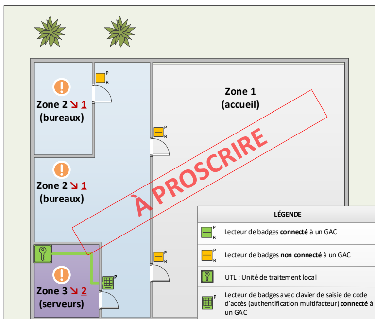
FIGURE 19 – Exemple d'architecture avec un contrôle d'accès physique sans gestion centralisée à proscrire
