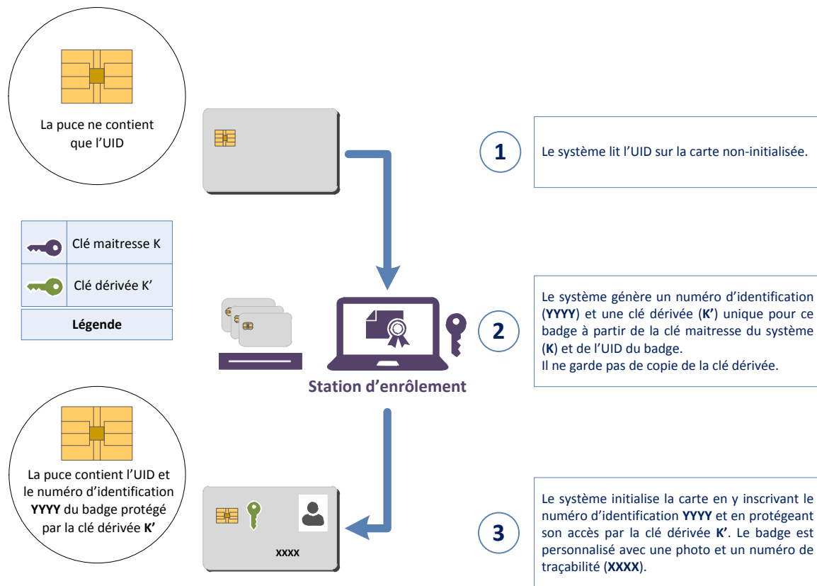
FIGURE 20 – Processus d'initialisation des badges à clé symétrique dérivée
