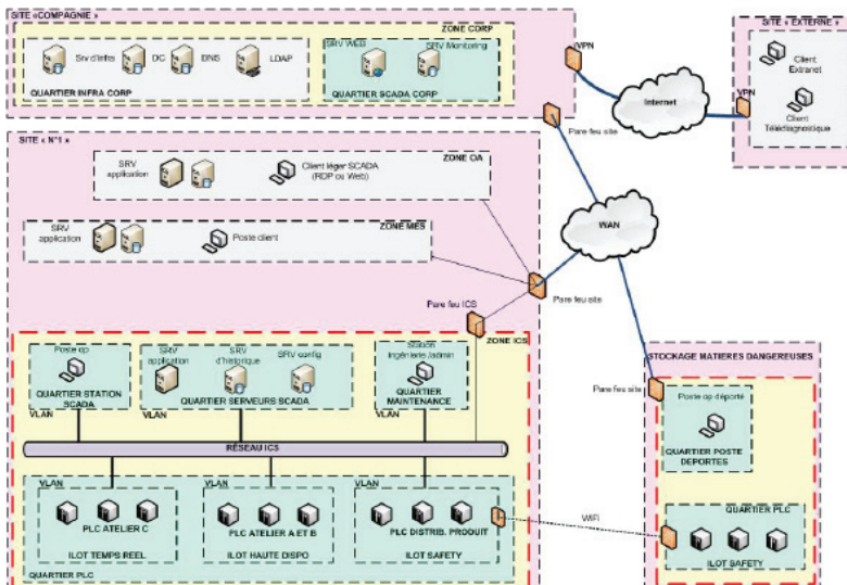
Fig. 4 - Proposition d'une architecture des installations industrielles et des interconnexions
