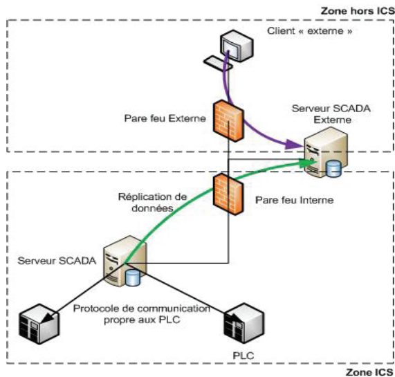
Fig. 8 - Accès au données SCADA au travers d'une zone démilitarisée : SECURISE
