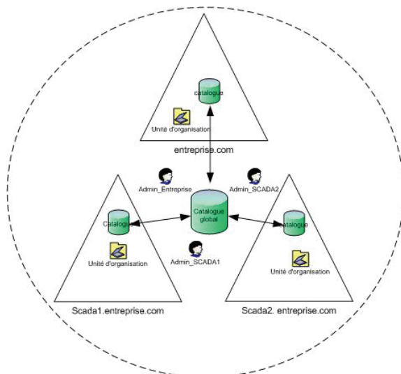
Fig 10 - Schéma de principe domaines et sous domaines
