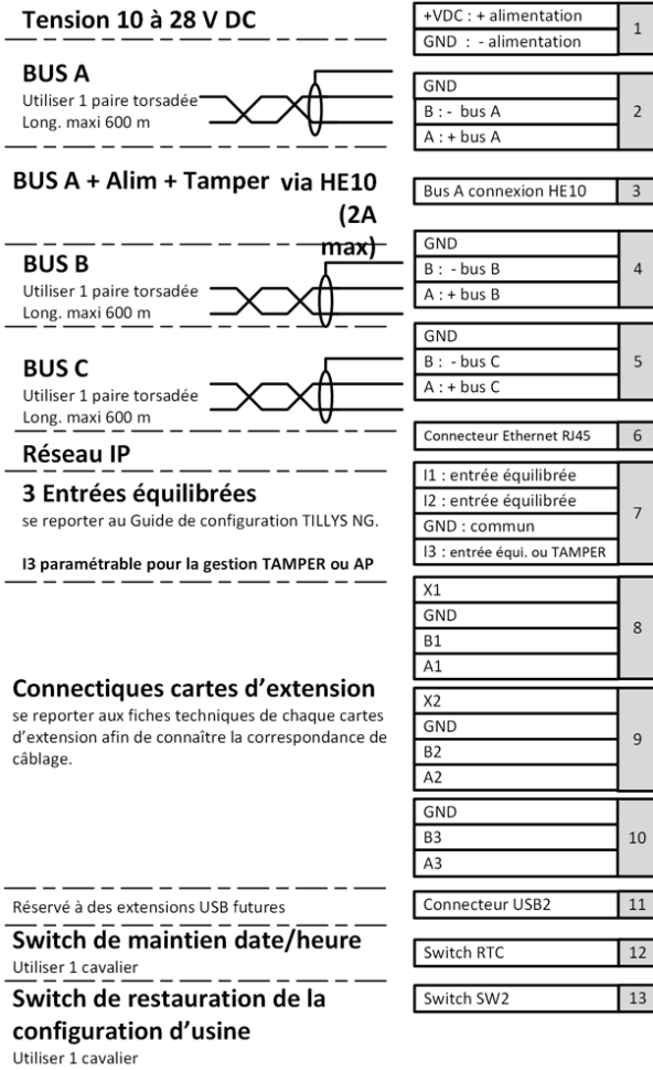
Figure 4 : Description matérielle module de base TILLYS-CUBE
