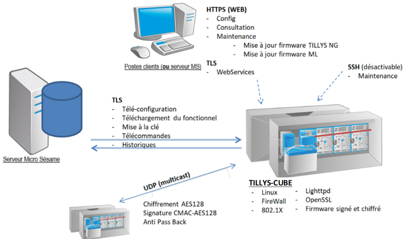
Figure 3 : Communication entre le serveur M.S et le coffret
