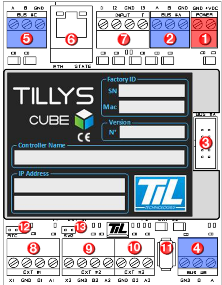
Figure 4 : Description matérielle module de base TILLYS-CUBE
