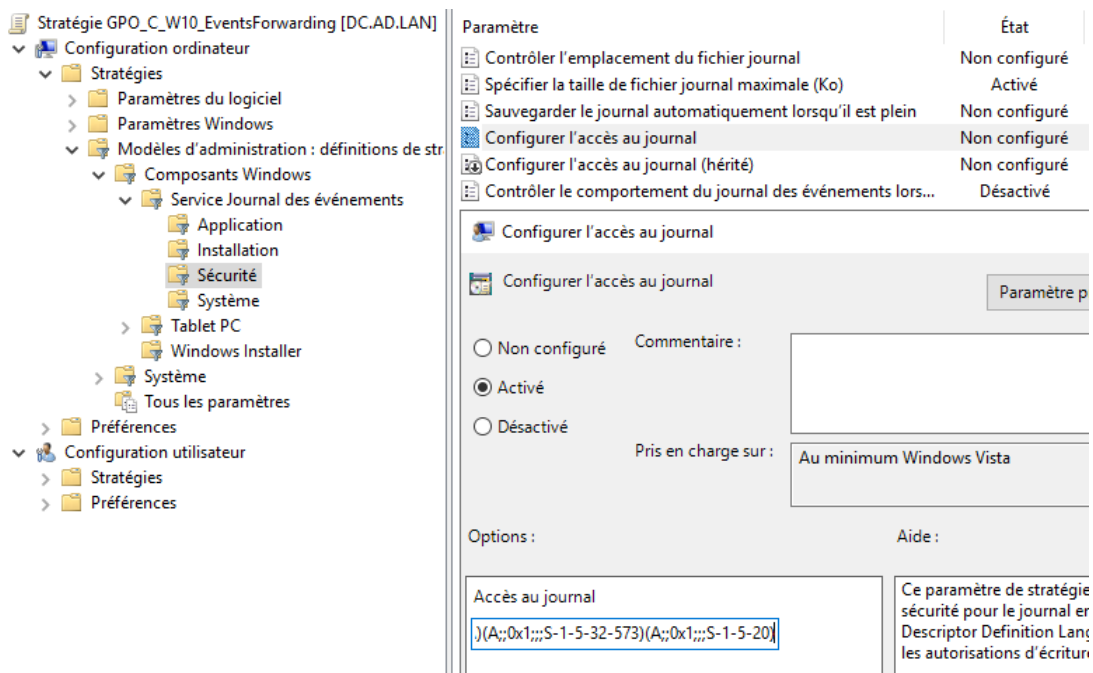
FIGURE 19 – Stratégie de configuration du descripteur de sécurité du journal Windows de sécurité
