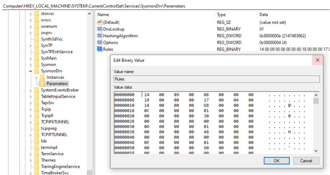
FIGURE 9 – Valeurs de clé de registre utilisées pour stocker la configuration de sysmon
