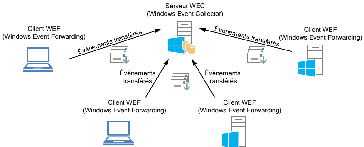
FIGURE 2 – Représentation de l'articulation entre WEC et WEF
