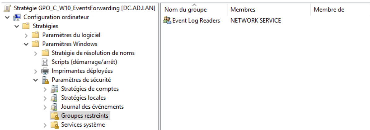
FIGURE 18 – Restriction de l'appartenance au groupe intégré Event Log Readers
