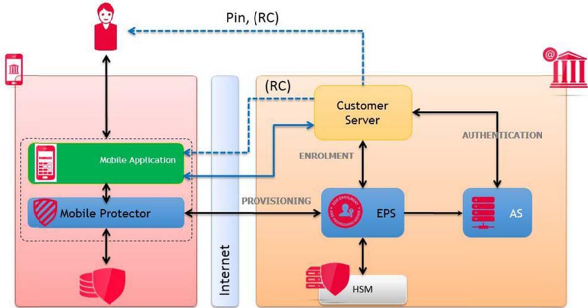
Figure 1 - Architecture Produit.
