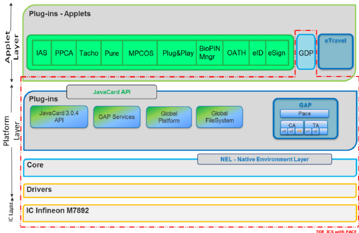
Figure 1 : Architecture du produit MultiApp V4.0.1 - PACE
