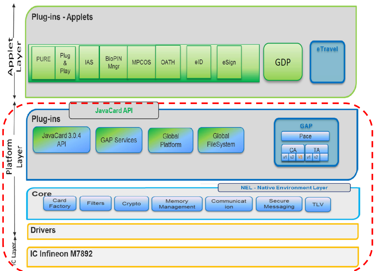
Figure 1 : Architecture du produit MultiApp V4
